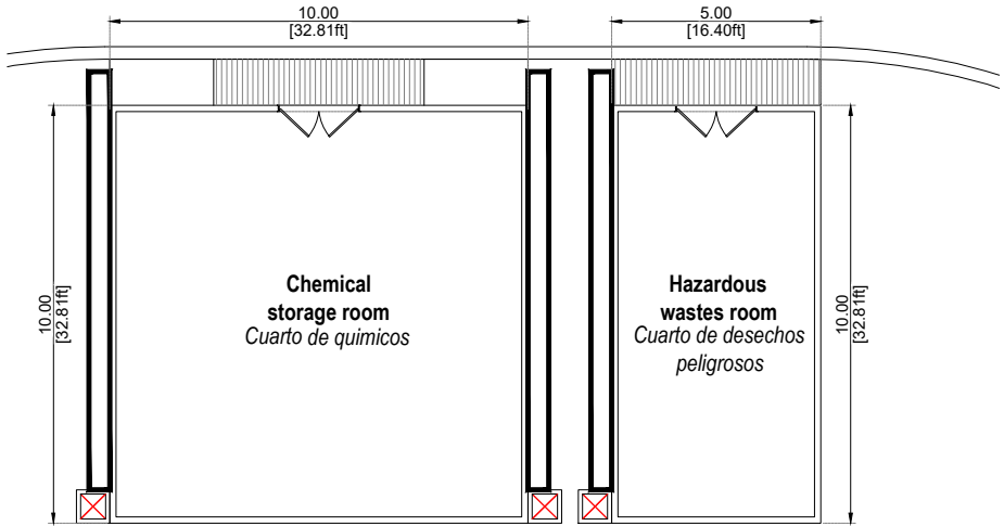
Chemical storage & Hazardous wastes rooms Cuarto de químicos y desechos peligrosos
