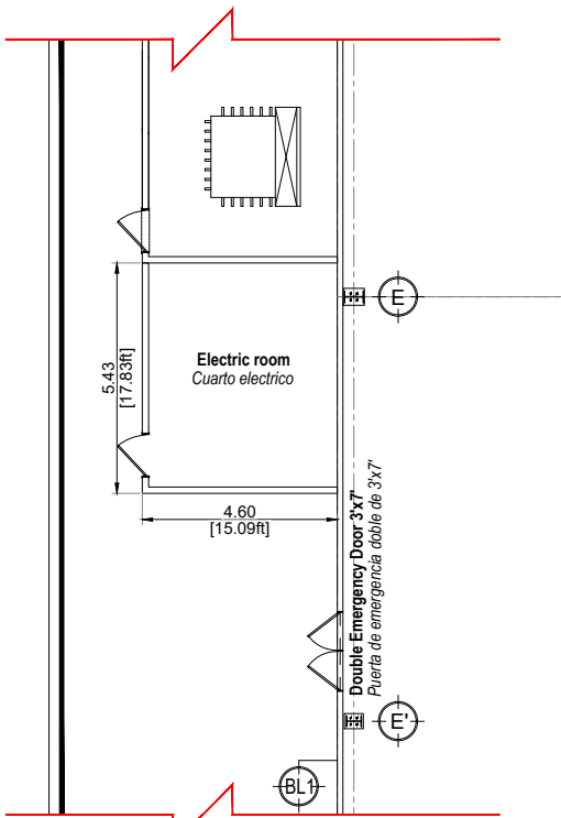
Electric room Cuarto eléctrico
